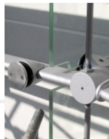
Detailansicht: Knoten, Glashalter, Riegel und Zugstäbe
